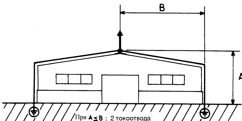
Фиг. 17. Брой на токоотводите
