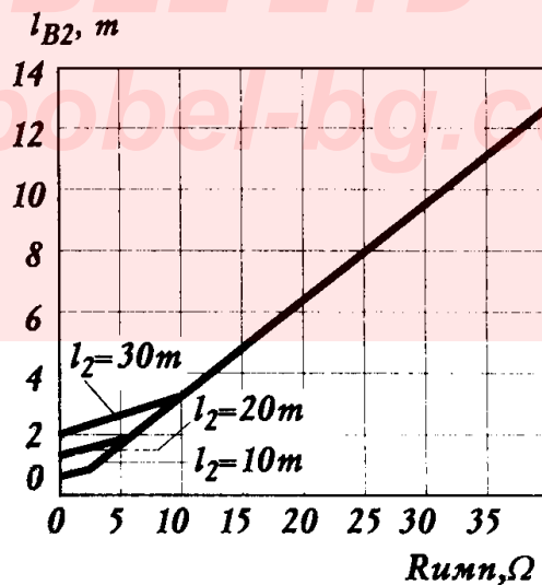
Фиг. 6. Минимални разстояния по въздуха между опората на мълниеотводното въже и защитавания обект, в зависимост от импулсното съпротивление на заземителя, за различни разчетни височини на опората: l_1 - разстояние между опорите на мълниеотводното въже - от 50 m до 200 m; l_1 - височина на опорите на мълниеотводното въже - 40 m; l_2 - разчетна височина на опората; l_{B2} - минимално разстояние по въздуха между опората на мълниеотводното въже и защитавания обект; R_{имп.} - импулсно съпротивление на заземителя
