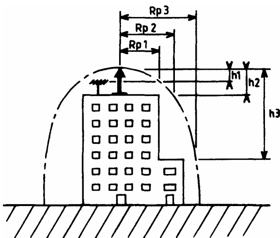
Фиг. 15. Радиуси на защита: h_n е височина на върха на мълниеприемника с изпреварващо действие по отношение на хоризонтална повърхност, преминаваща през върха на разглеждания защитаван обект; R_{pn} - радиус на защита на мълниеприемника с изпреварващо действие за разглежданата височина
