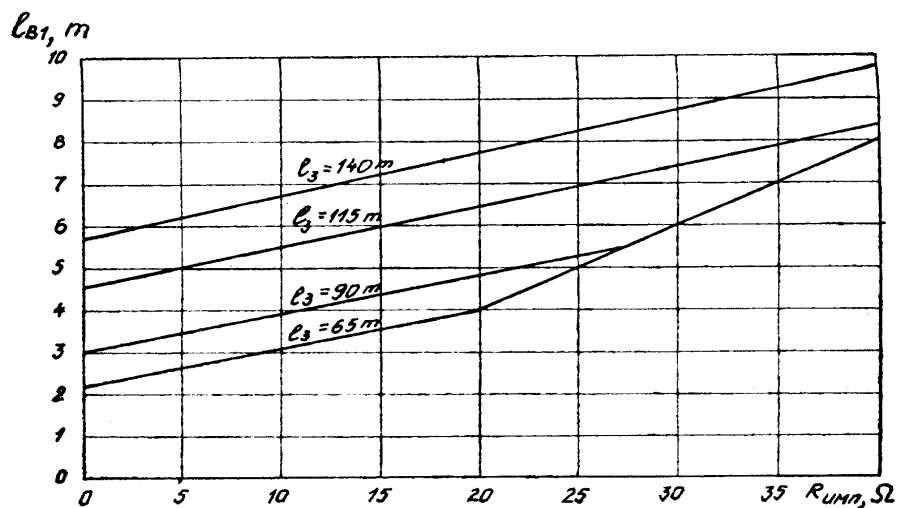
Фиг. 5. Минимални разстояния по въздуха между мълниеотводното въже и защитавания обект, в зависимост от импулсното съпротивление на заземителя, за различни разчетни дължини на мълниеотвода: l_{B1} - минимално разстояние по въздуха между мълниеотводното въже и защитавания обект; l_3 - разчетна дължина на мълниеотвода; R_{имп.} - импулсно съпротивление на заземителя
