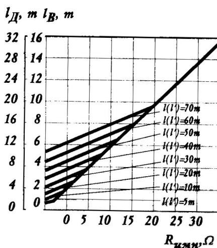
Фиг. 3. Минимални разстояния между токоотвода и защитавания обект и минимална дължина на електроизолационната опора на мълниеотвода, в зависимост от импулсното съпротивление на заземителя, за различни разчетни дължини на мълниеотвода: l_b - минимално разстояние по въздуха между мълниеотвода и защитавания обект; l_d - минимална дължина на електроизолационната опора на мълниеотвода; l и l' - разчетна дължина на мълниеотвода; R_{имп.} - импулсно съпротивление на заземителя
