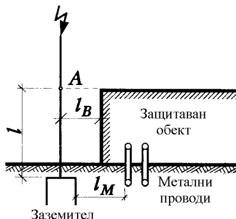
Фиг. 1. Мълниезащита чрез отделностоящ прътов мълниеотвод: А - точка от мълниеотвода, съответстваща на най-високата част на защитавания обект; l - разчетна дължина на мълниеотвода; l_B - минимално разстояние по въздуха между мълниеотвода и защитавания обект; l_M - минимално разстояние между заземителя и подземните метални проводни
